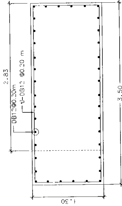
แบบขยายตอม่อ มาตราส่วน 1:30
