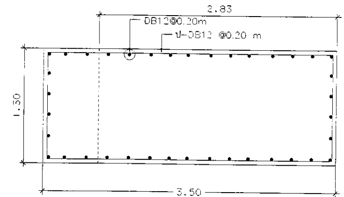
แบบขยายตอม่อ
