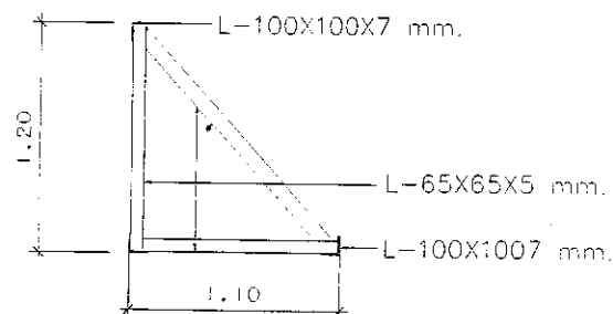
แบบขยายคาน RB1
