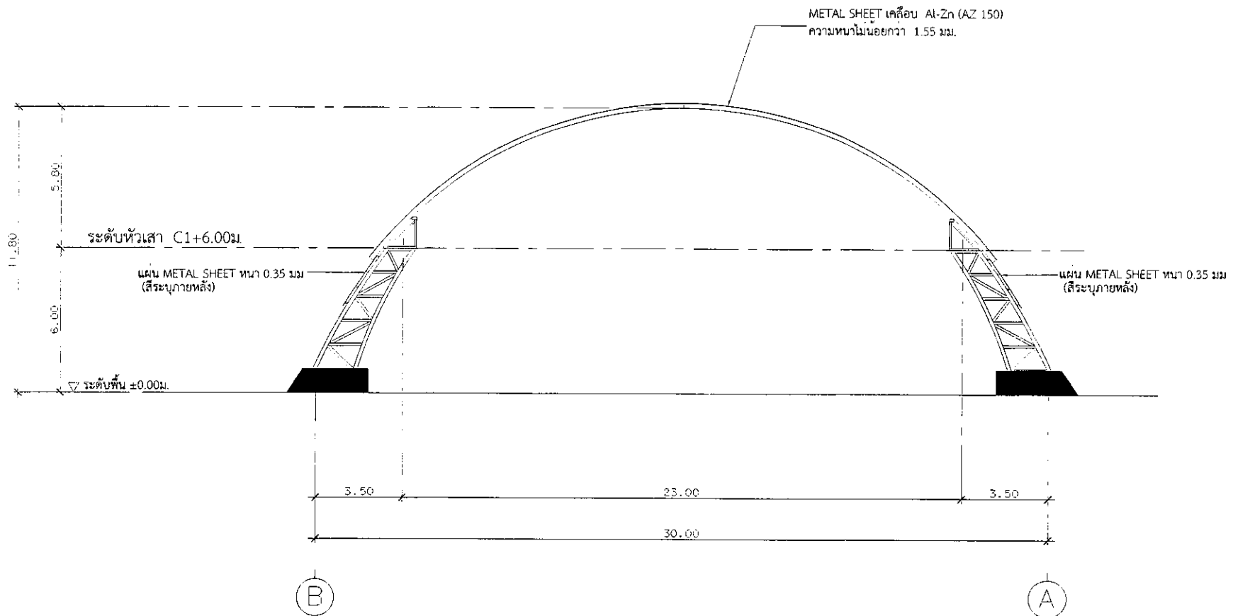
รูปด้าน C
