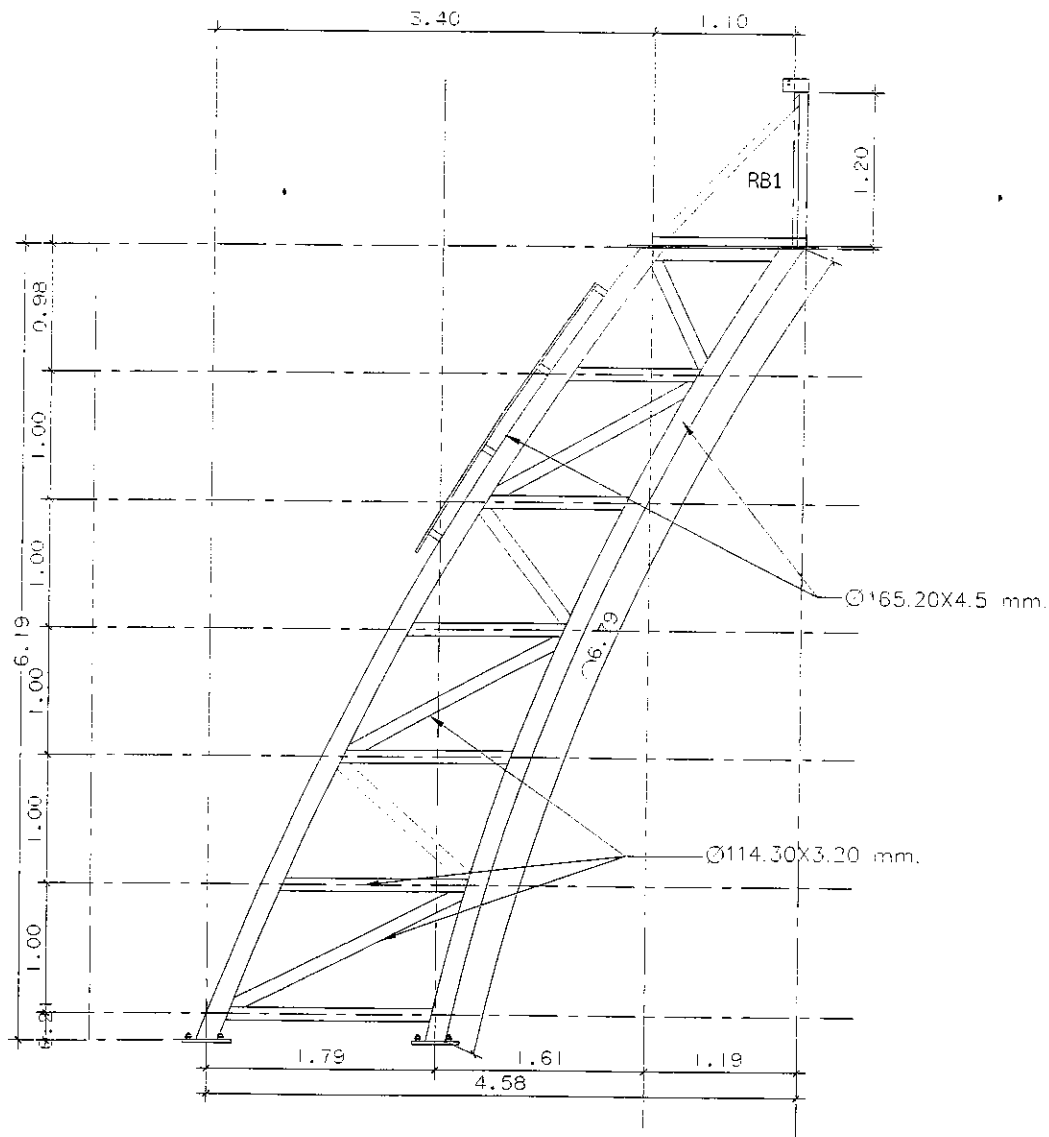
แบบขยายเสา C1
