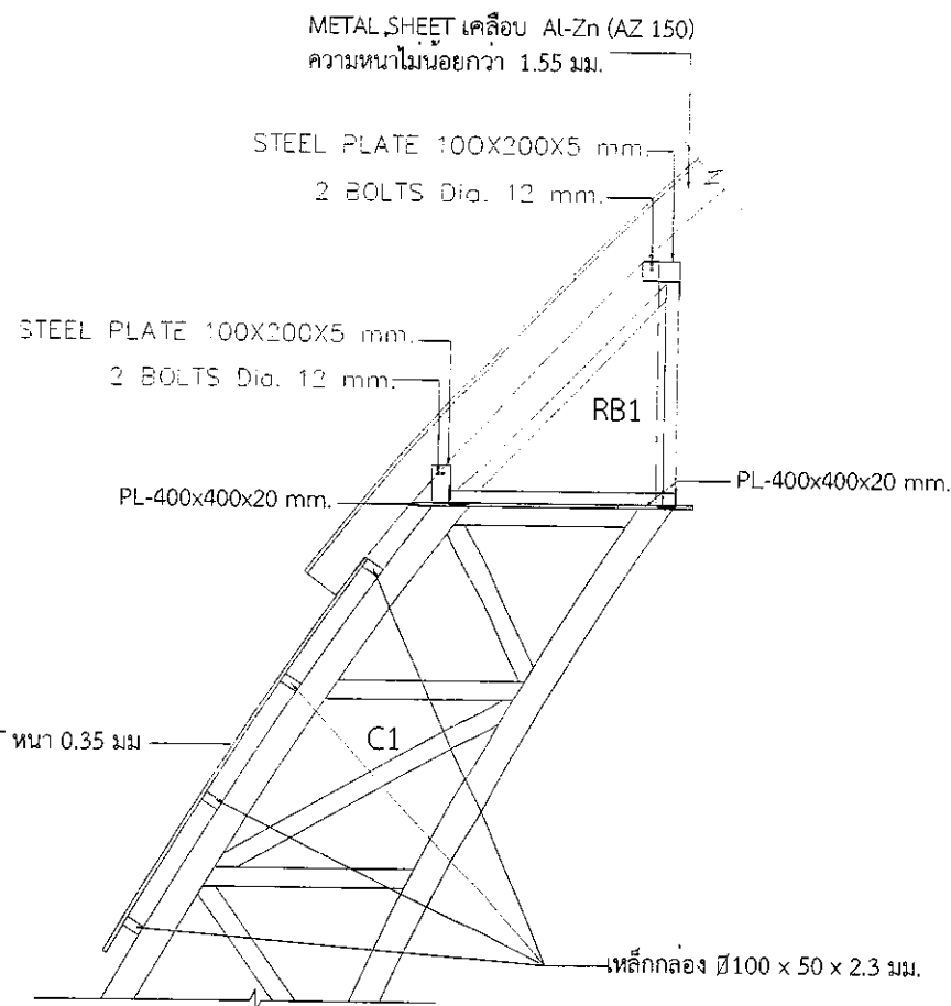
แบบขยาย 1
