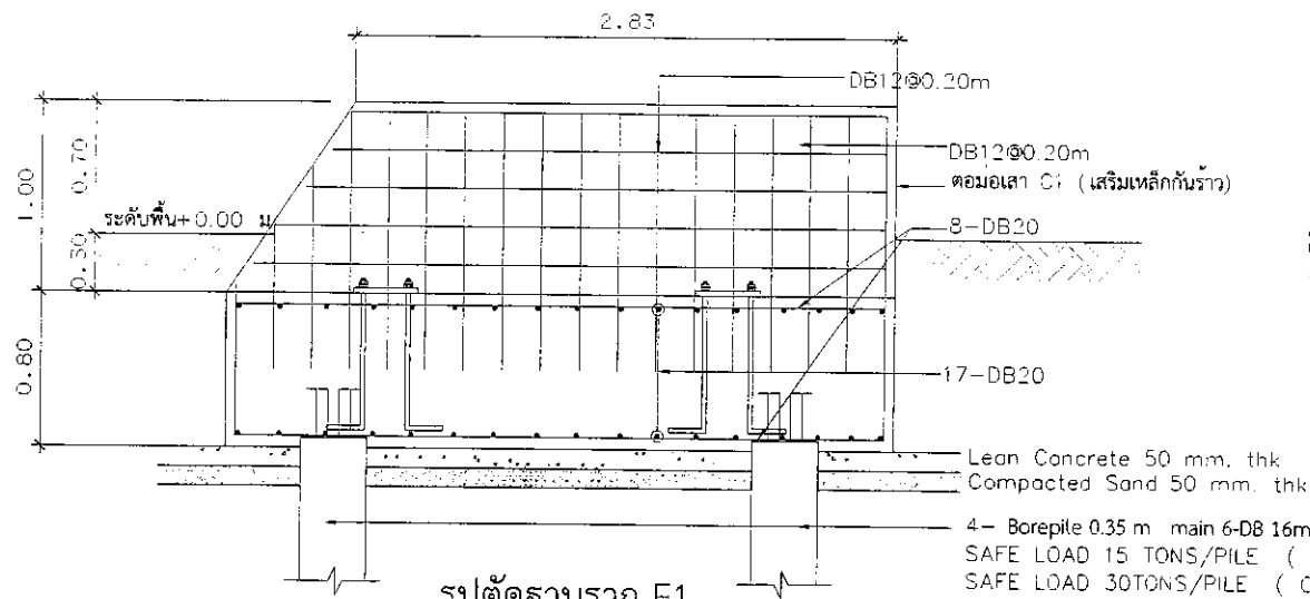
รูปตัดฐานราก F1
