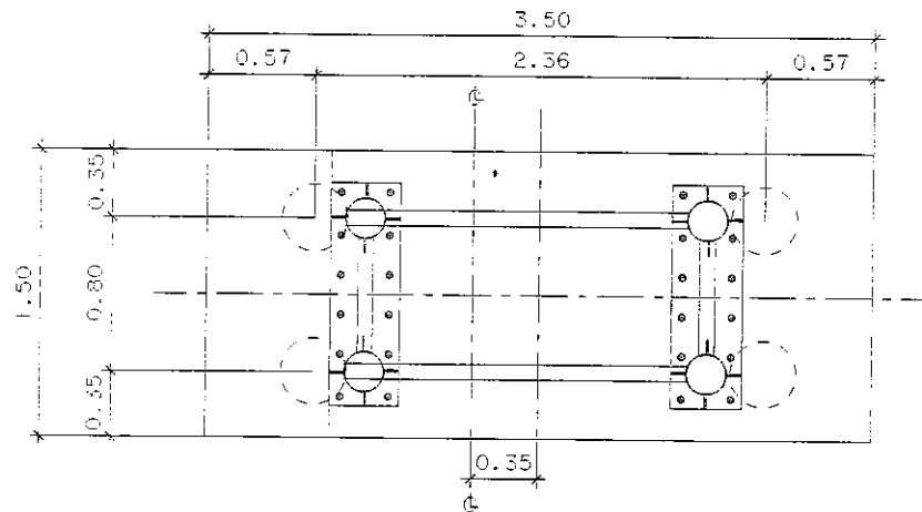
แปลนฐานราก F1
