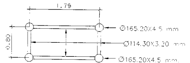
แบบขยายเสา C1 เริ่ม
